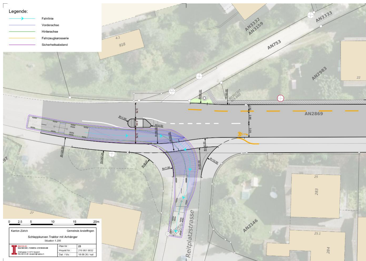
Abbildung 32: Schleppkurve Traktor mit Anhänger (Landstrasse dorfauswärts > Reitplatzstrasse)
