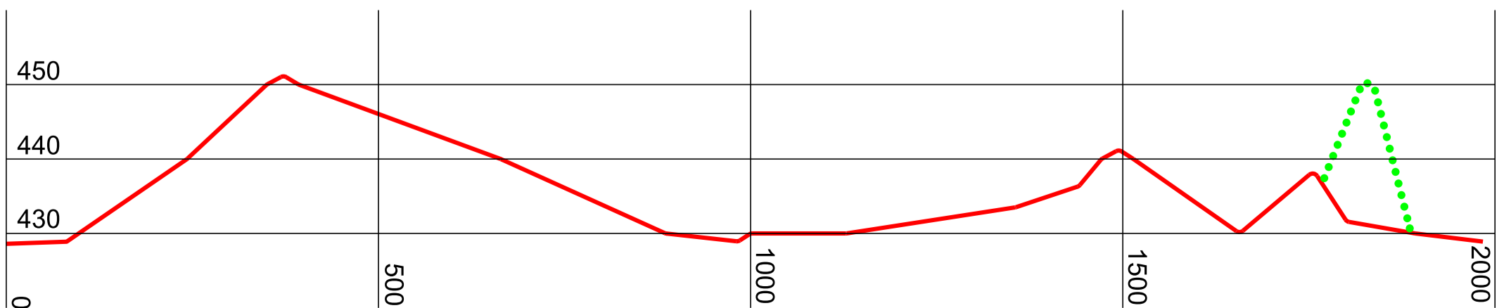
Längenprofil 10-fach überhöht
